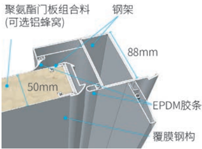
ISMART-S 系列断面展示
