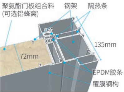
ISMART-L 系列断面展示
