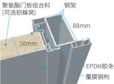
ISMART-V 系列断面展示
